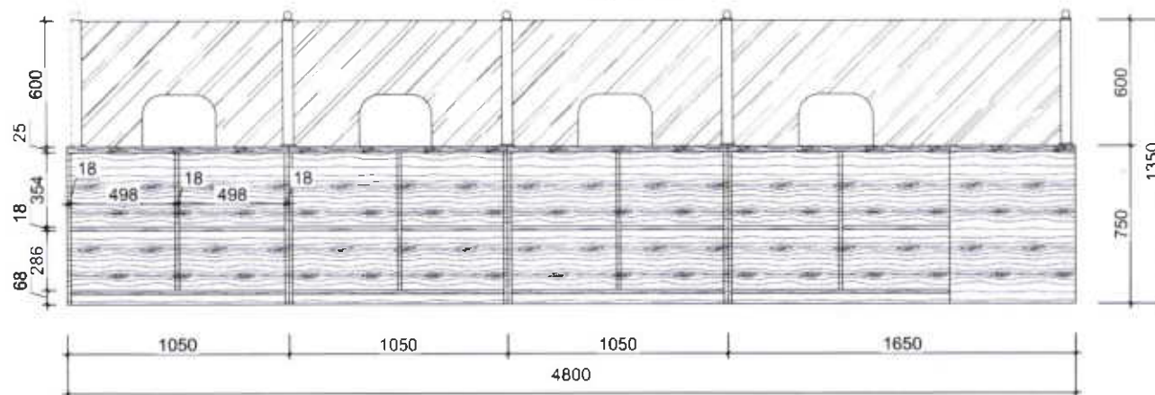
MẶT ĐỪNG TRONG
