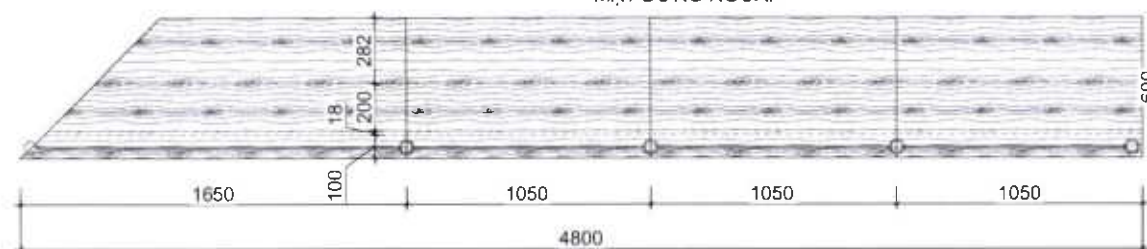
MẶT BẰNG
