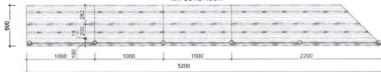
MẶT BẰNG
