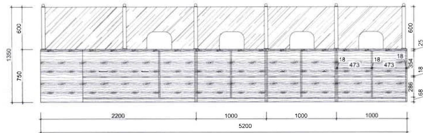
MẶT ĐỨNG TRONG
