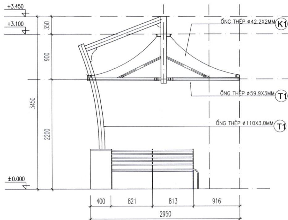
MẶT ĐỨNG KHUNG KẾT CẤU MÁI SỐ 02 TL:1/40
