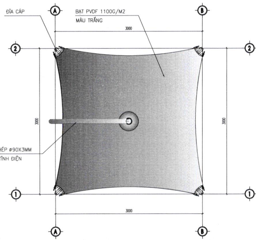
MẶT BẰNG MÁI PVDF MÁI CHE 02 TL:1/50
