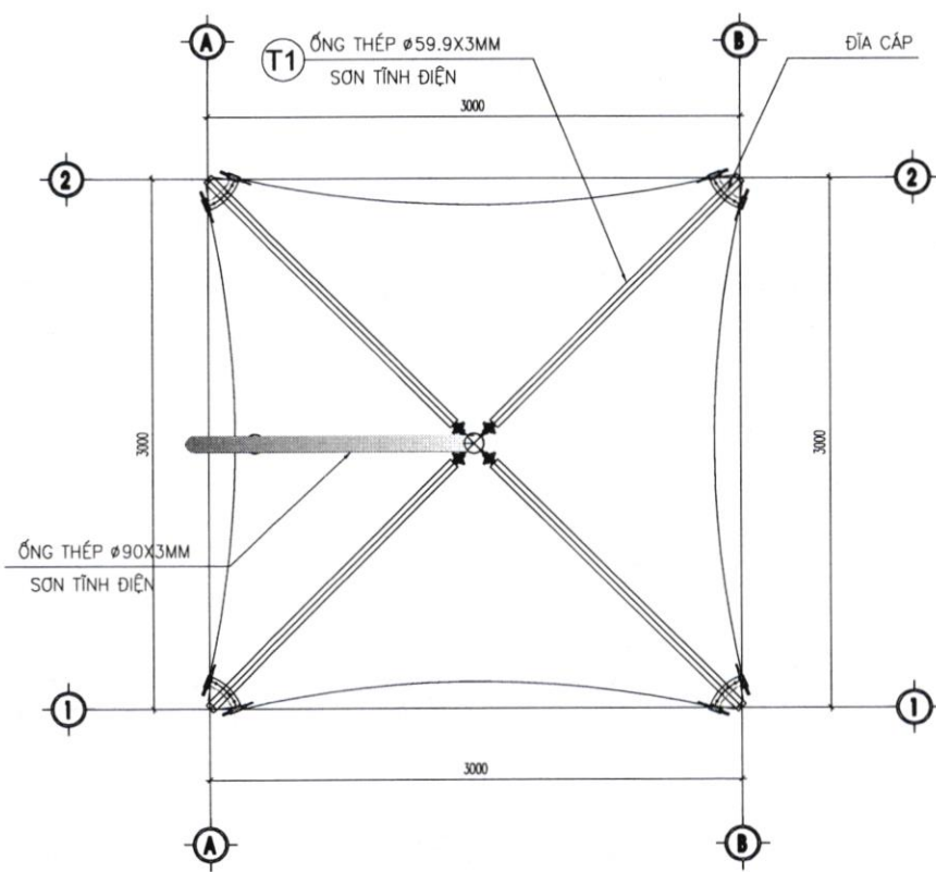
MẶT BẰNG KHUNG Ô CHE 02 TL:1/50
