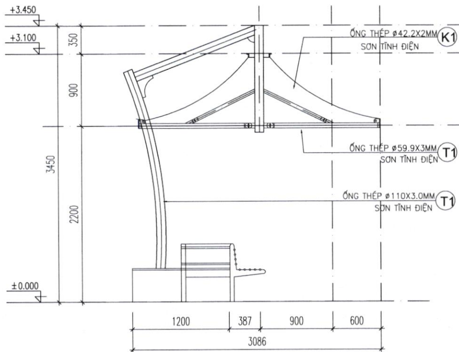
MẶT ĐỪNG KHUNG KẾT CẤU MÁI SỐ 02 TL:1/40
